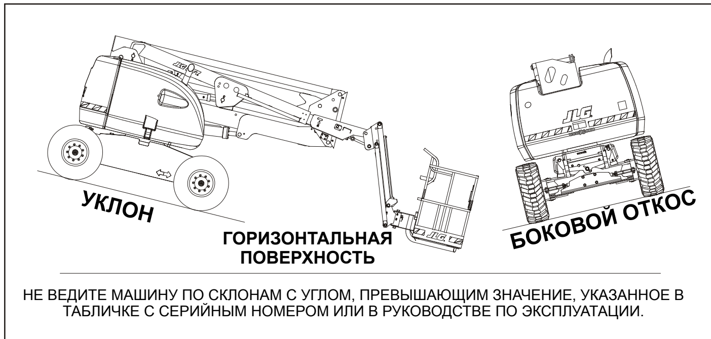
Рис. 4-3. Уклон и боковые откосы
